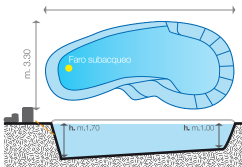
Pianta e sezione Sirio 720
