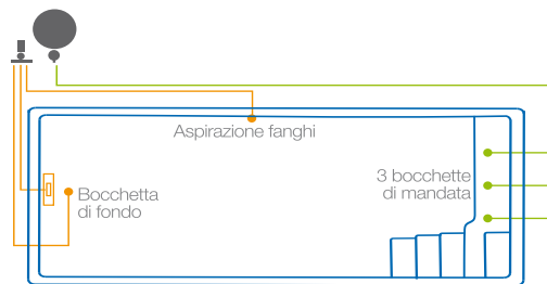
Schema dei flussi
