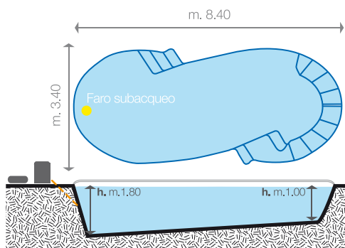
Pianta e sezione
