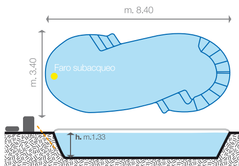
Pianta e sezione Antares
