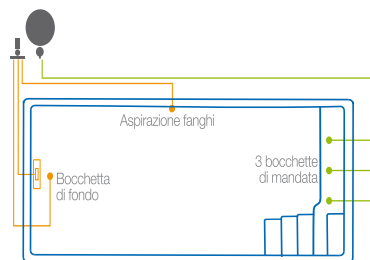
Schema dei flussi
