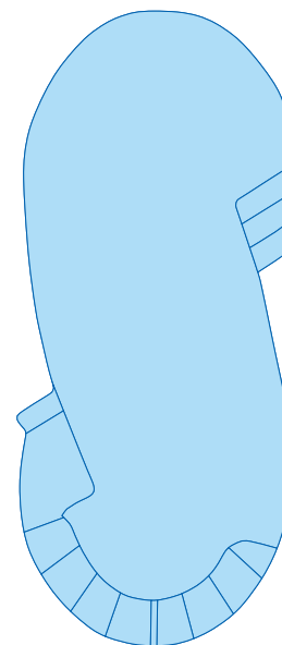
Antares
