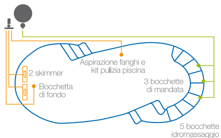
Schema dei flussi
