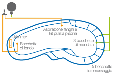
Schema dei flussi
